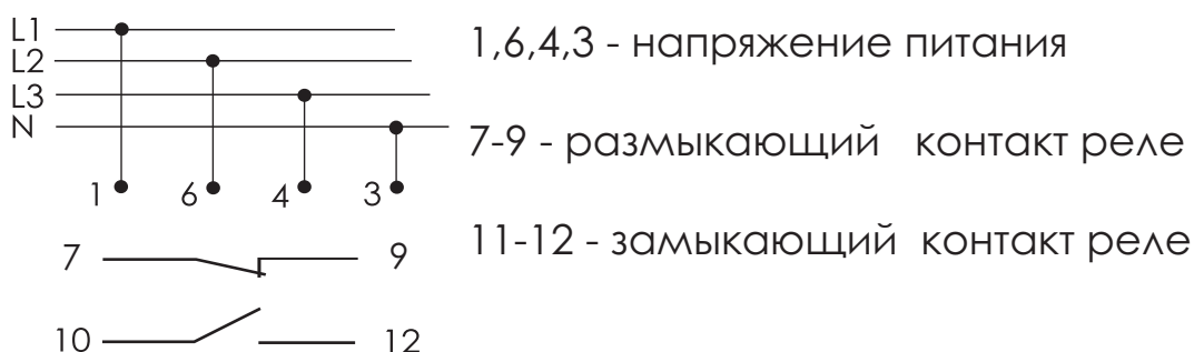
Рис.2 Назначение контактов.
